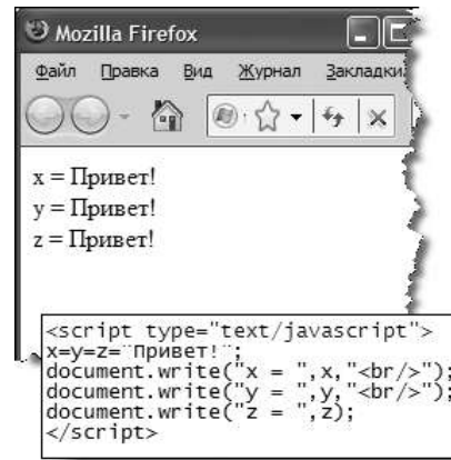
Рис. 16.12. Каскадное использование оператора присваивания значения сразу нескольким переменным
