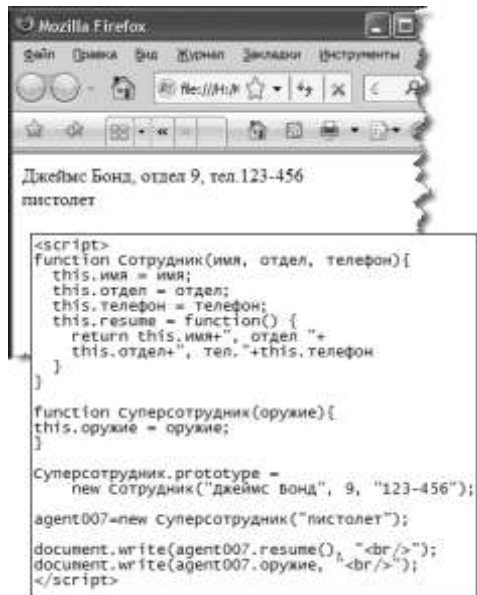
Рис. 16.23. Пример наследования свойств объекта через прототип
